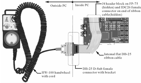
图 2 手轮与 FP-75 板的连接
