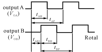
图 5 输出波形图
