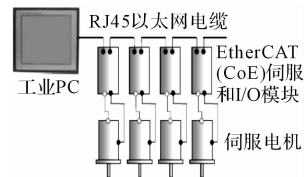
图 1 EtherCAT 通讯平台结构图
