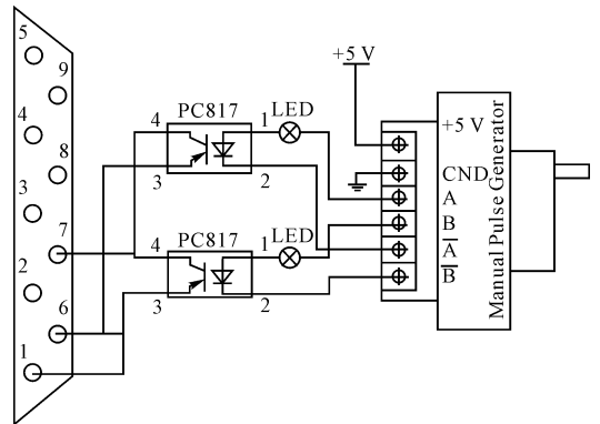
图 6 转换电路图
