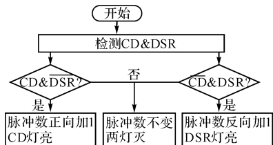
图7 测试程序流程图
